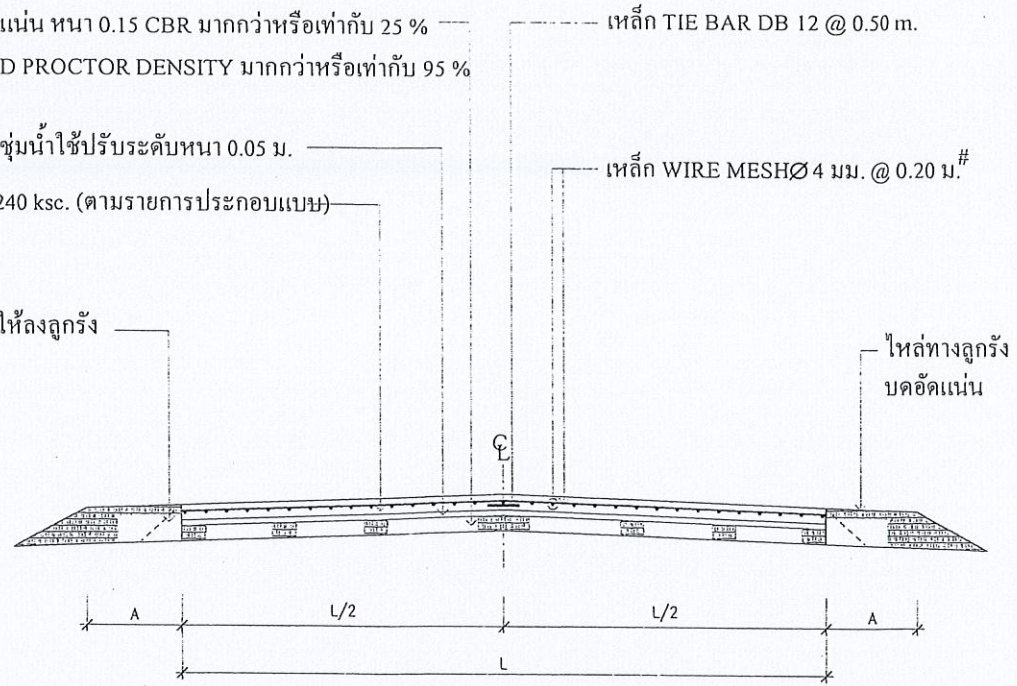
รูปตัดตามขวางถนน
