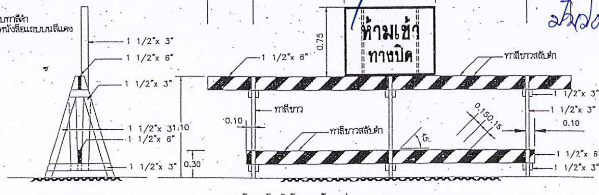
แผงกั้นทำด้วยไม้ และป้ายเครื่องหมายจราจร หมายเลข 4
