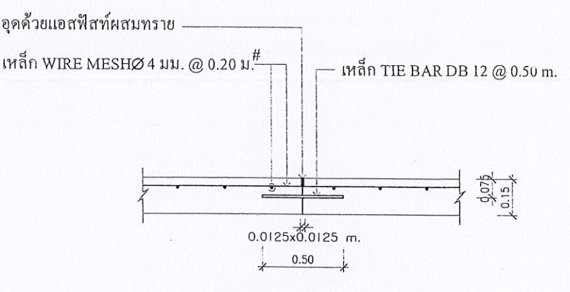
LONGITUDINAL JOINT
