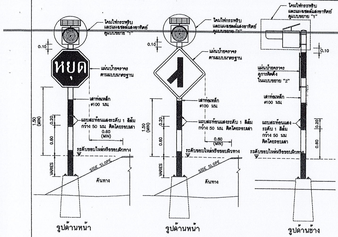
แสดงการติดตั้งสัญญาณไฟกระพริบร่วมกับป้ายบังคับหรือป้ายเตือน (เสาเหล็ก) ไม่แสดงมาตราส่วน
