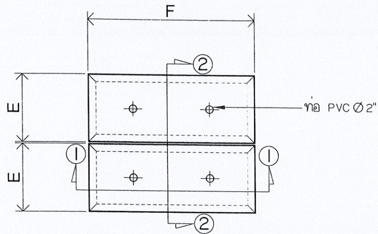
แปลนฝาบ่อพักในผิวจราจร มาตรฐาน 1:25
