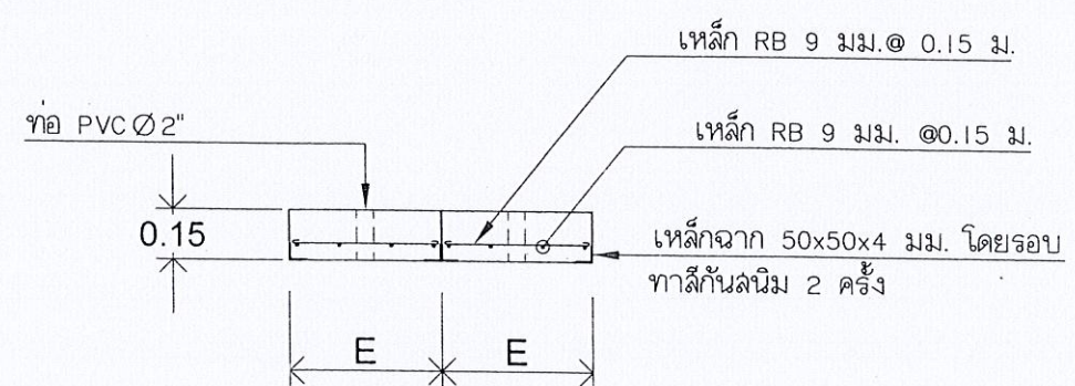
รูปตัด 2 มาตรฐาน 1:25
