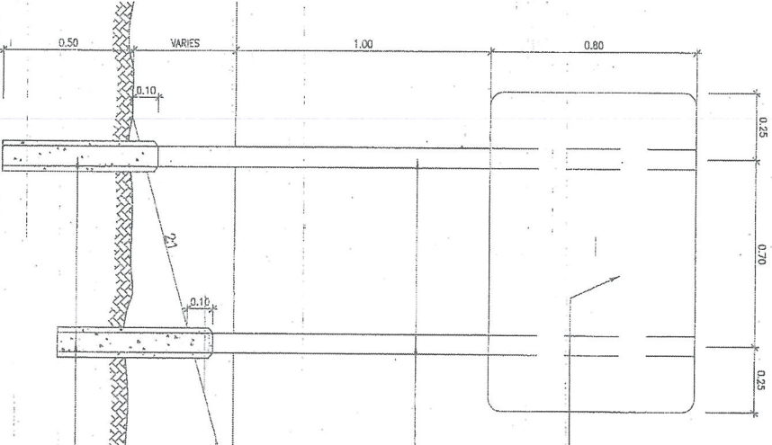
ติดตั้งการปักเสาป้าย
