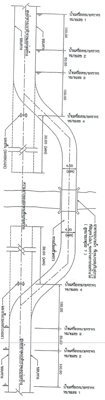
แบบแปลนหน้าทางของทางไปเมือง และส่วนหน้าซึ่งตั้งกับบ้นร่องจราจร
