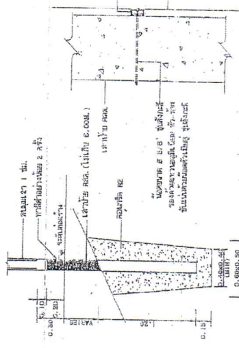
แสดงการฝังสายไฟ
