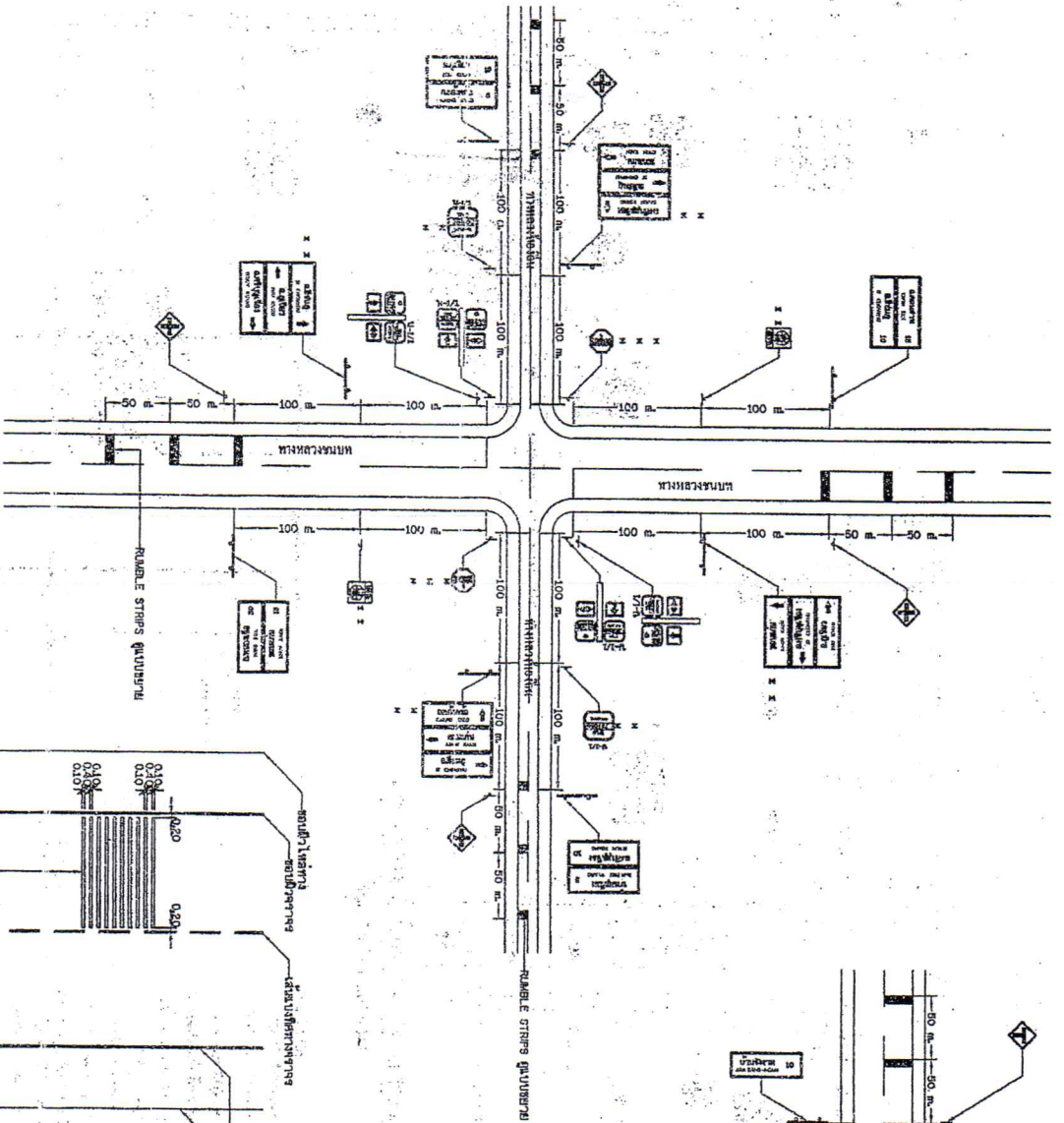
แผนผังการติดตั้งป้ายจราจรบริเวณสี่แยก ( เชื่อมทางหลวงชนบท )
