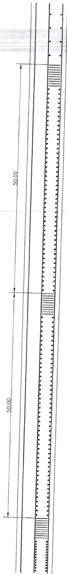
แบบขยายเส้นชะลอความเร็วช่วง B มาตราส่วน NOT TO SCALE
