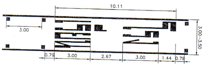
ตัดขวาง "โรงเรียน" บนผิวทาง ขนาดจราจร NOT TO SCALE
