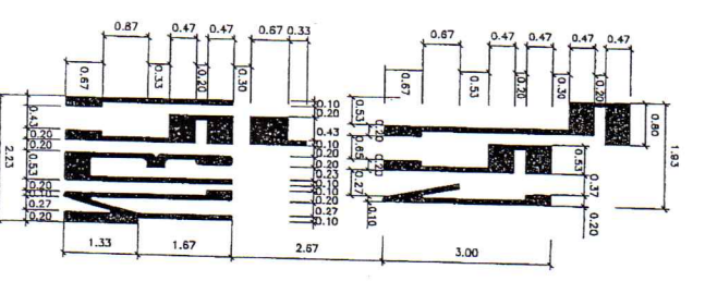
ตัดขวาง "โรงเรียน" บนผิวทาง ขนาดจราจร NOT TO SCALE
