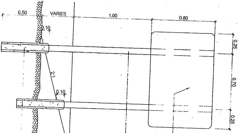
แสดงการปักเสาปูน
