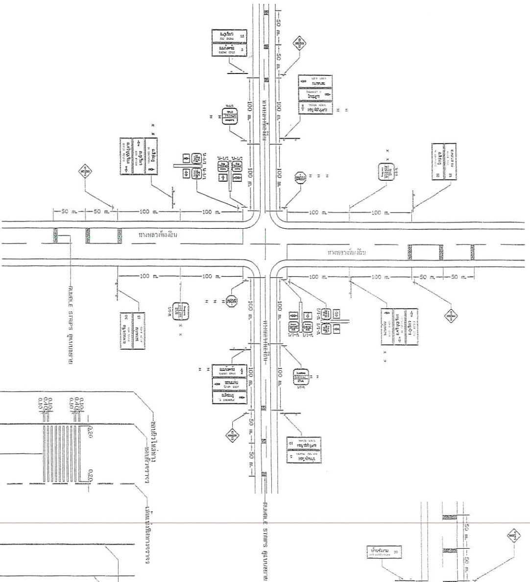
แผนผังการติดตั้งป้ายจราจรควบคุมสัญญาณไฟจราจร ( ใช้ช่องทางการจราจรสองทิศทาง )
