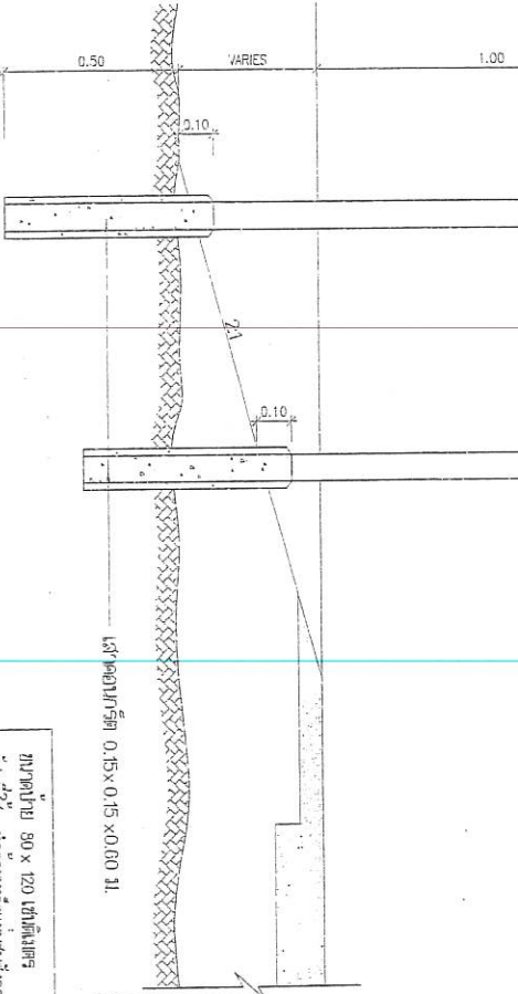
แผ่นดัดการปักเสาป้าย
