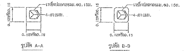
รูปตัดเสาป้าย (ดูทฤษฎีเหตุ ข้อ 4)
