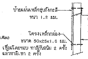
แสดงการติดตั้งป้ายแนะนำ
