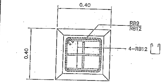
รูปตัด (ข)
