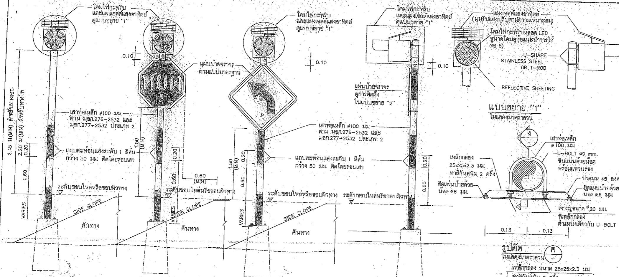
ไฟกะพริบ
