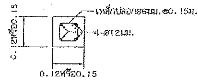
รูปลัด A-A
