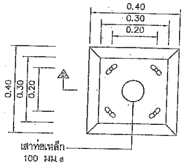
แปลน
