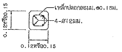
รูปลัด B-B
