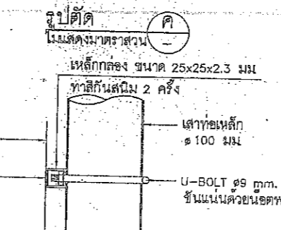
รูปตัด (ค)
