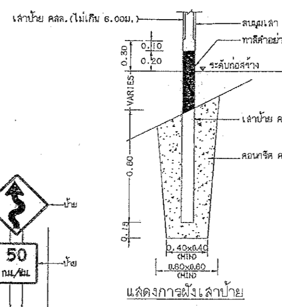
แสดงการปักเสาป้ายแนะนำ น-1 และ น-4
