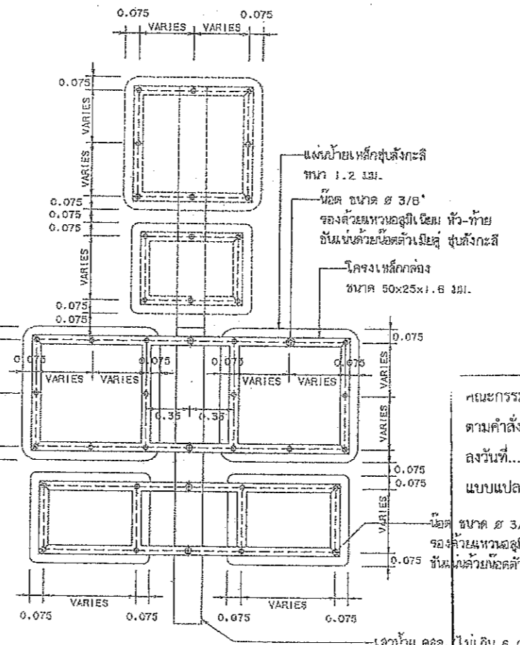
แสดงการยึดโครงป้ายชุดระบุทิศทาง
