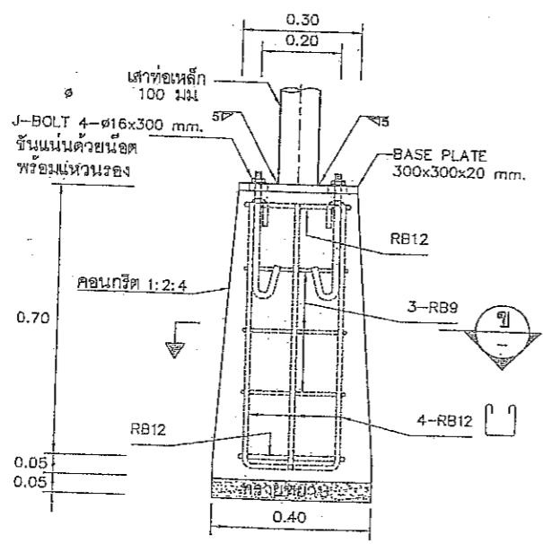
รูปตัด (ก)
